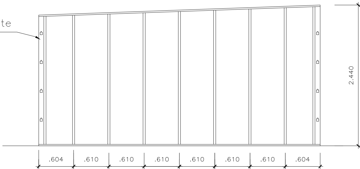
ELEVACION LATERAL IZQUIERDA
